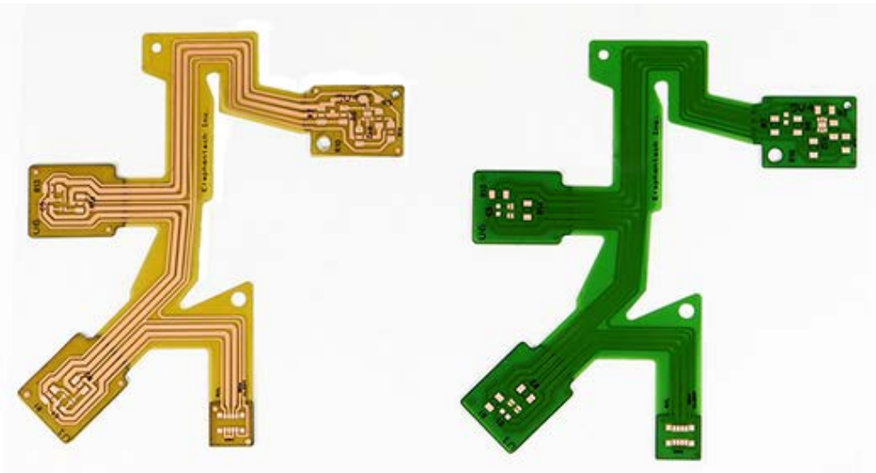
左：P-Flex™ PI 透明阻焊剂（另有 白·黑可选 需另外收取费用）
